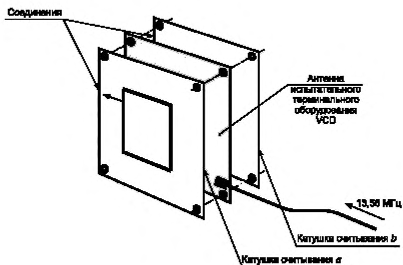
Рисунок С.2 — Катушки считывания в сборе
