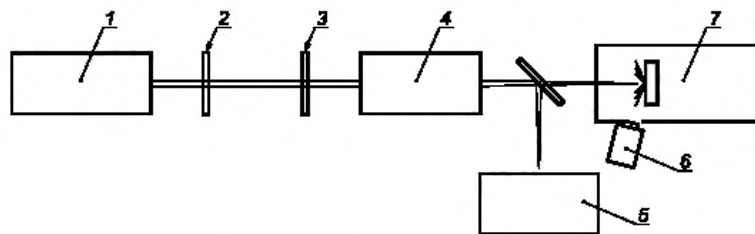
1 — лазерная система; 2 — переменный аттенуатор; 3 — фазовая пластинка; 4 — фокусирующая система; 5 — блок диагностики пучка; 6 — система онлайн-обнаружения разрушения; 7 — отсек для образцов
