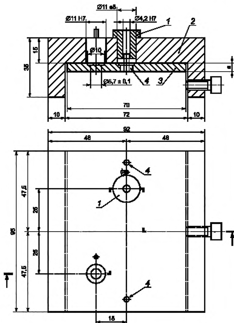
1 — втулка для сверления с шаблоном; 2 — шаблон для сверления; 3 — фрикционная пластина; 4 — центрирующий штифт. a — толщина в зависимости от необходимой глубины проникновения
