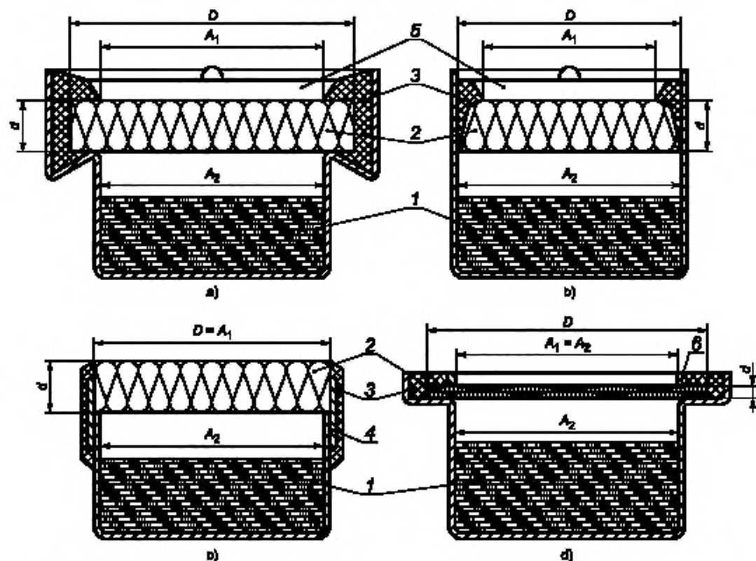
Типы испытательных чашек
