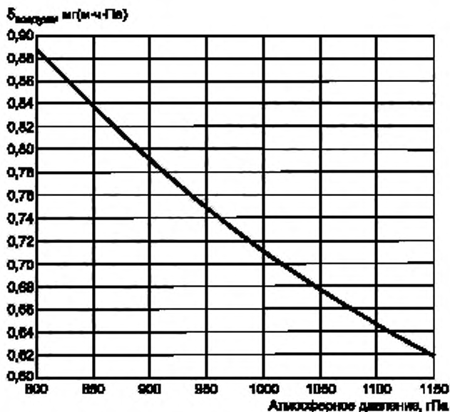
Рисунок 1 — Паропроницаемость воздуха при 23 °C
