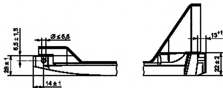
Рисунок 4 — Подошва для испытаний формы Т с вырезом для позиции вставки
