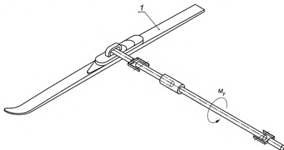
1 — неподвижно закрепленная лыжа
