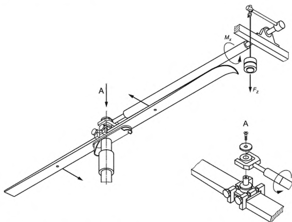
Рисунок 11 — Испытание отсоединения с комбинированной нагрузкой для влияния нагрузки при крене
