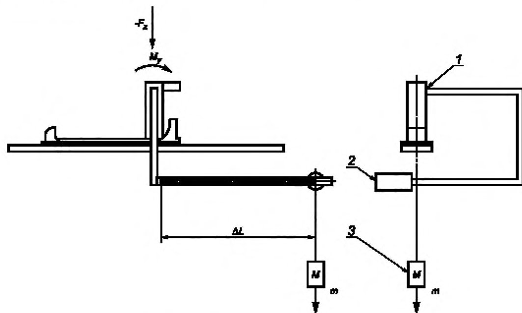
t — момент и сила; 2 — уравновешивающая масса; 3 — дополнительная масса
