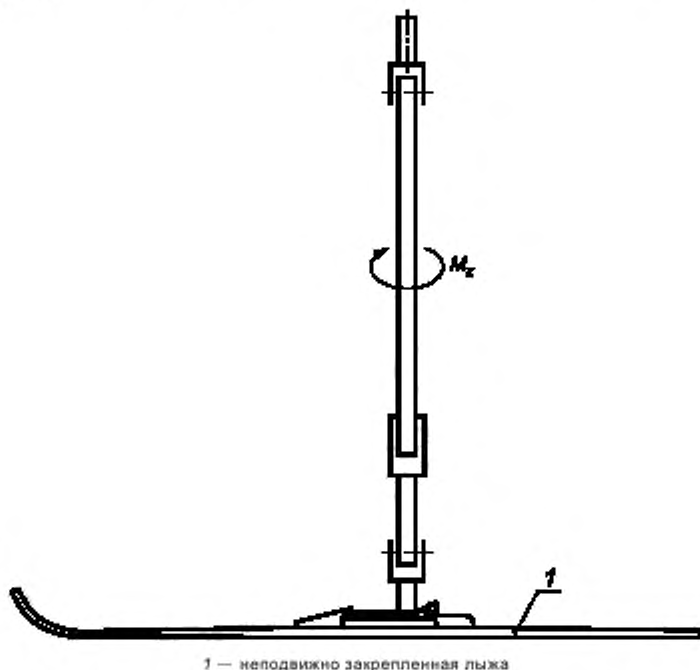
Рисунок 1 — Приложение крутящего момента M_x и измерение M_{x\max}
