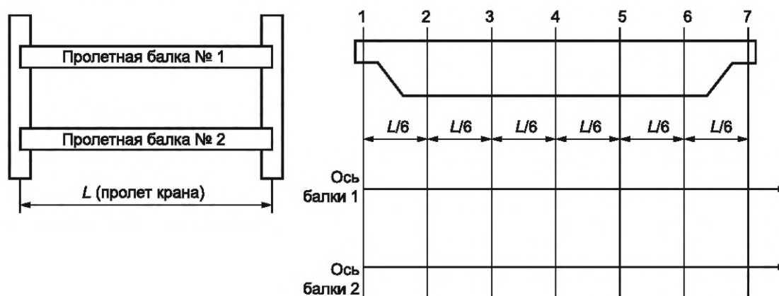
Рисунок И.1 — Схема измерений высотного положения пролетных балок мостов крана и планово-высотной съёмки рельсового пути грузовой тележки
