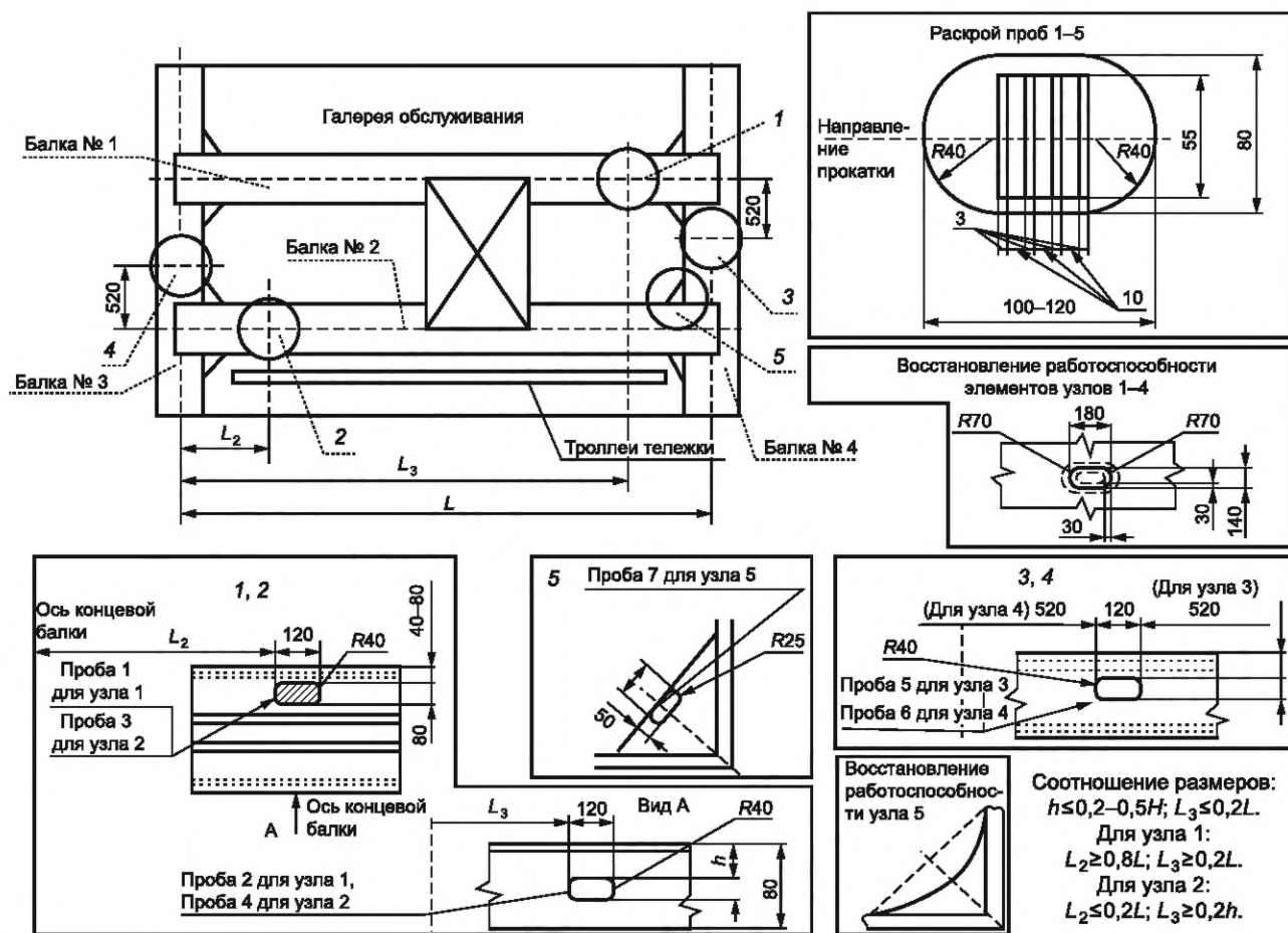
Рисунок Т.1 — Схема отбора проб на мостовых кранах с балками коробчатой конструкции
