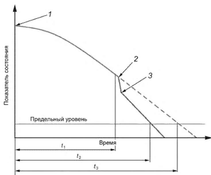
1 — начальное значение ПС; 2 и 3 — моменты изменения траектории старения под ВВФ проектной аварии и поставочных окружающих условий
