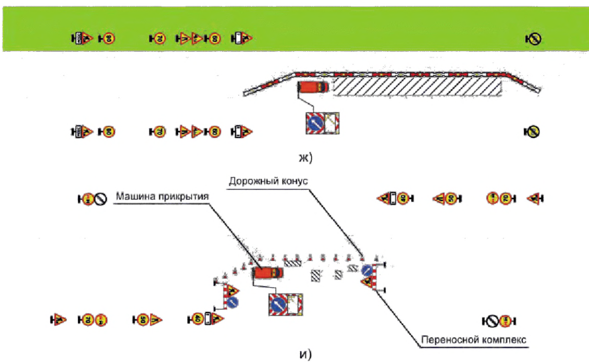
Рисунок Ж.1, лист 3
