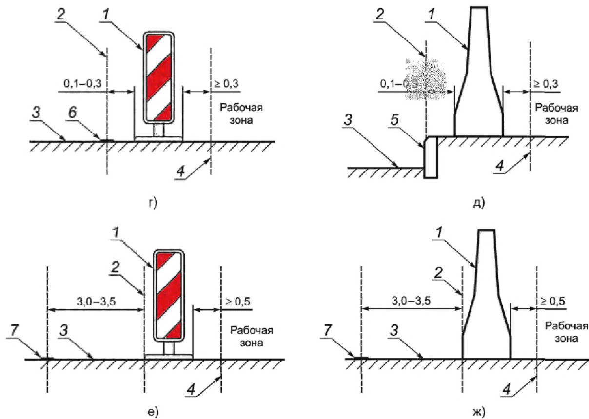
Рисунок Б.1, лист 2
