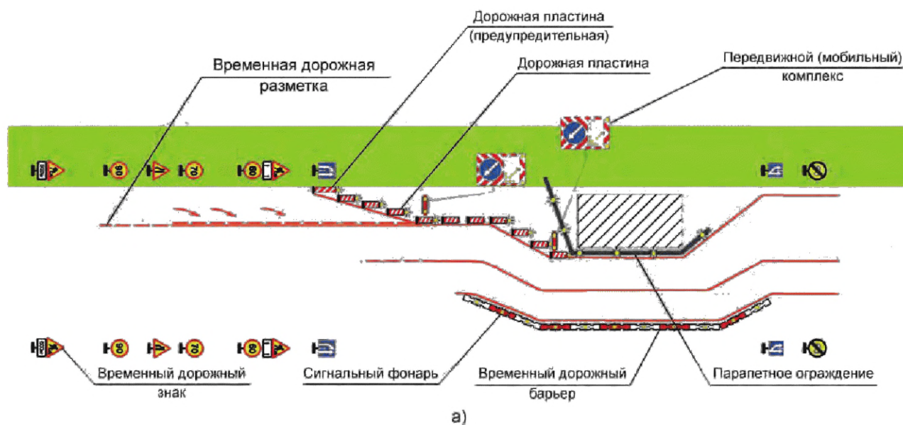
Рисунок Ж.1, лист 1 — Примеры применения временных технических средств организации дорожного движения:
