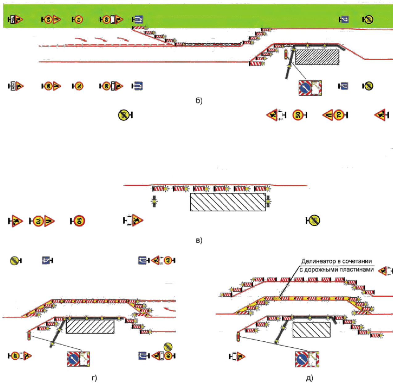
Рисунок Ж.1, лист 2
