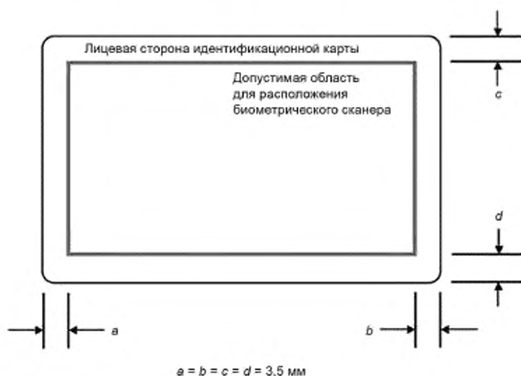
Рисунок 1 — Допустимая область для расположения биометрического сканера на лицевой стороне идентификационной карты
