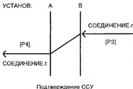
Рисунок 6 Установление ССУ, подфаза «подтверждение ССУ»
