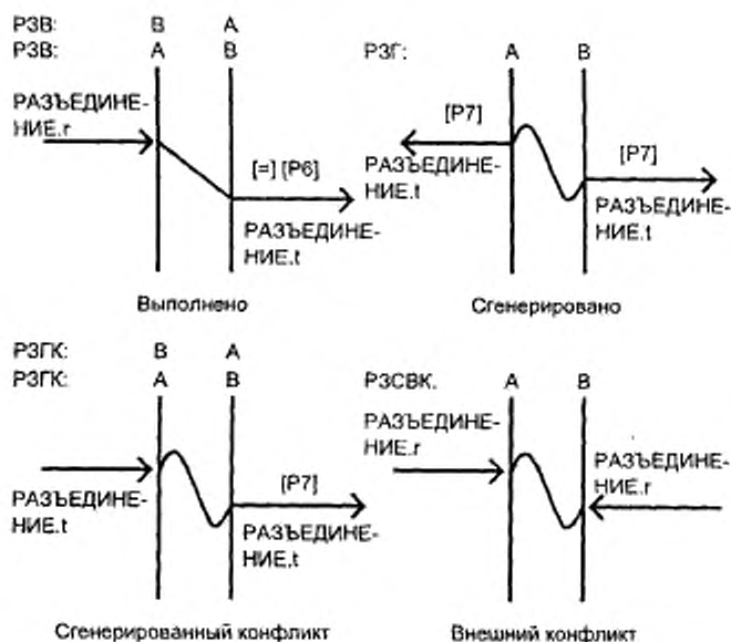
Рисунок 9 — Фаза «разъединение ССУ»
