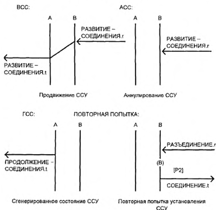
Рисунок 5 — Установление ССУ, подфаза «развитие ССУ»
