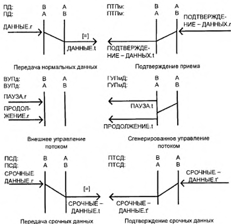
Рисунок 7 — Передача данных, подфаза «передача»
