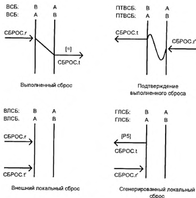
Рисунок 8 — Передача данных, подфаза «сброс»
