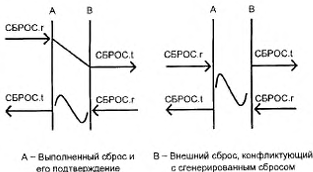
Рисунок 13 — Примеры базового сброса
