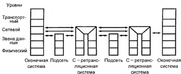
А — Полная архитектурная модель (ИСО 8448)
