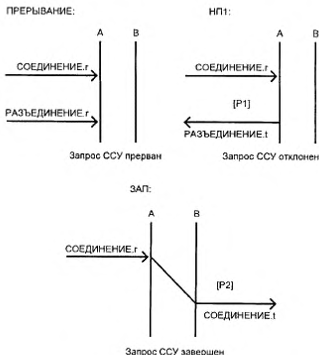
Рисунок 4 — Установление CSU, подфаза «запрос CSU»
