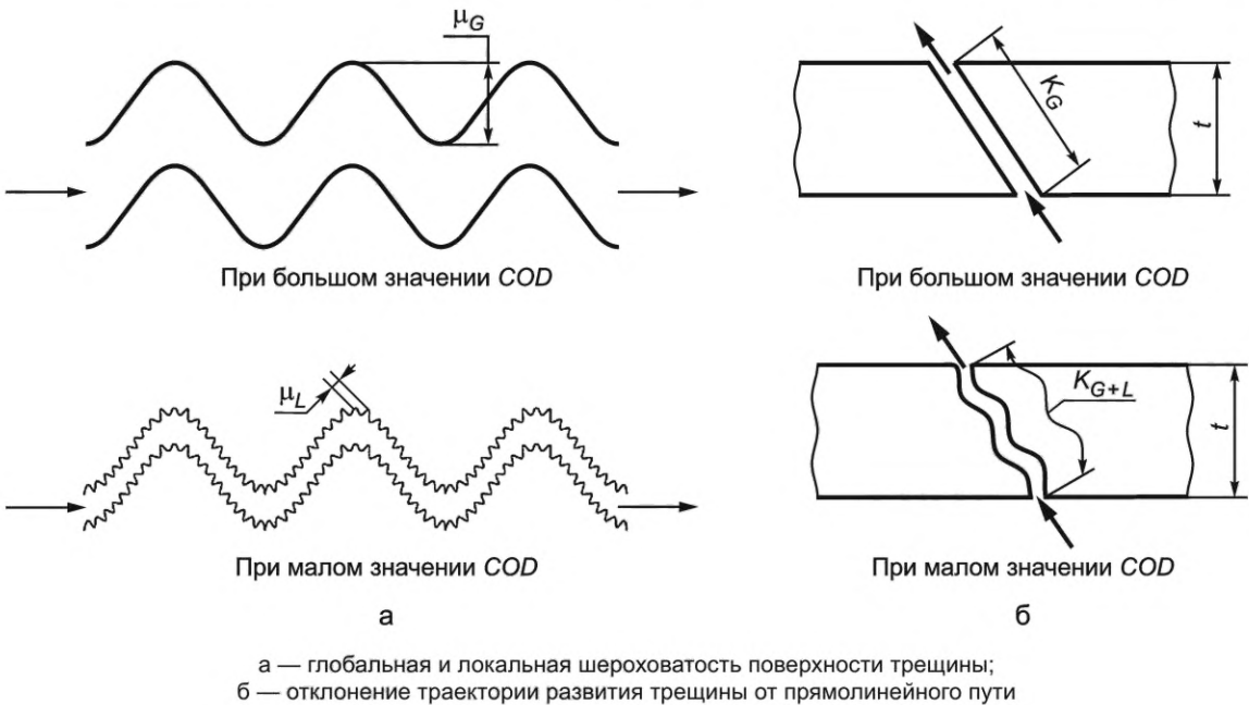
Рисунок Е.1 — Схематичное изображение морфологии трещины
