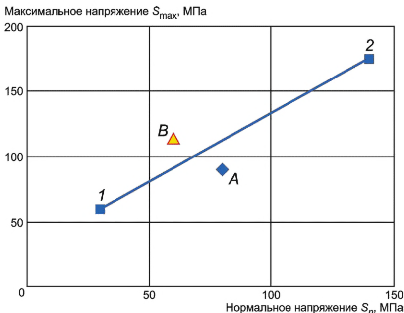
Рисунок Ж.1 — Линейная аппроксимация типичной ГРК
