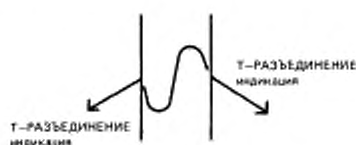
Разъединение СТУ по инициативе поставщика УТУ
