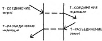
Отклонение пользователем УТУ запроса на установление СТУ
