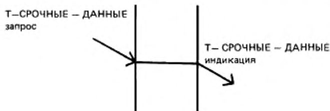
Рисунок 7 — Последовательность примитивов при успешной передаче срочных данных
