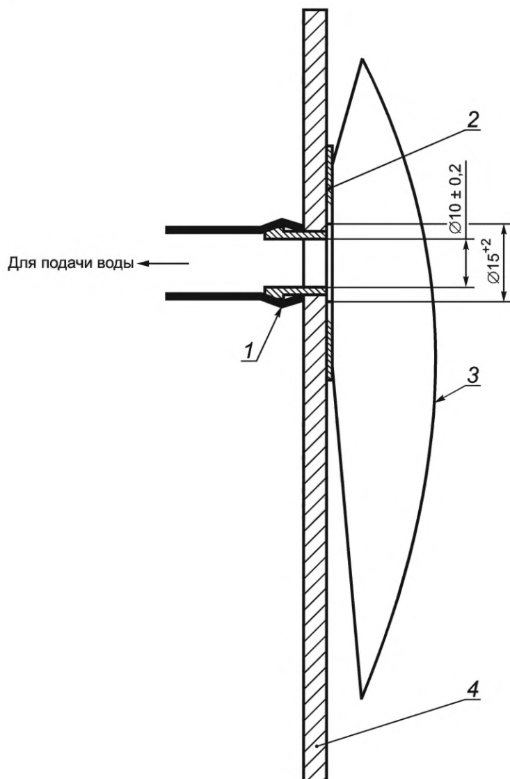
Рисунок 8 — Размещение для измерения испытательного объема
