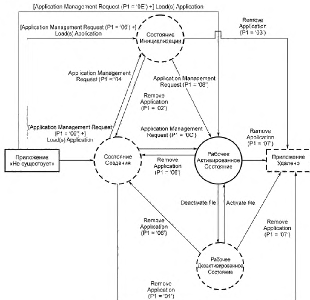
Рисунок 2 — Диаграмма жизненного цикла приложения
