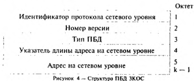
Рисунок 4 — Структура ПБД ЗКОС
