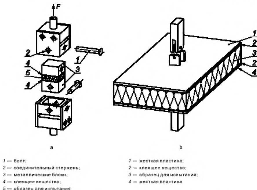
Рисунок 1 — Примеры приспособлений для крепления образца
