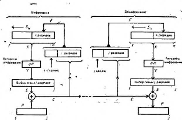
Рисунок 2 — Режим работы шифрования с обратной связью (CFB)
