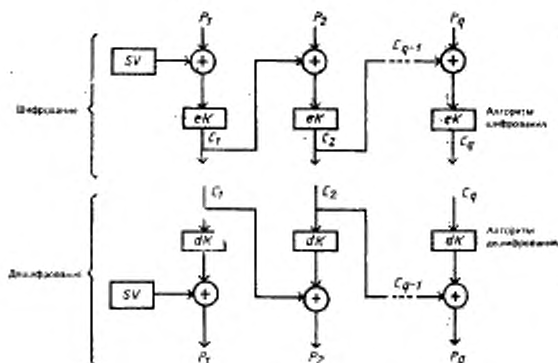
Рисунок 1 — Режим работы последовательного блочного шифрования (СВС)
