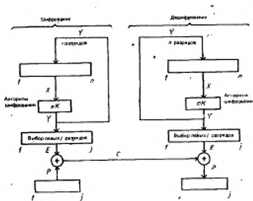
Рисунок 3 — Режим работы шифрования с обратной связью по выходу (OFB)
