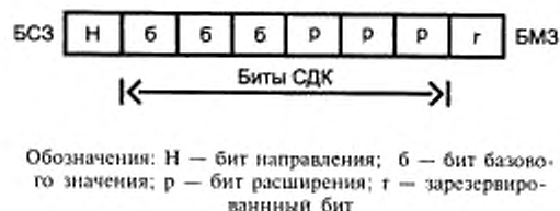
Рисунок С.4 — Базовые биты и биты расширения области СДК второго октета поля УМ
