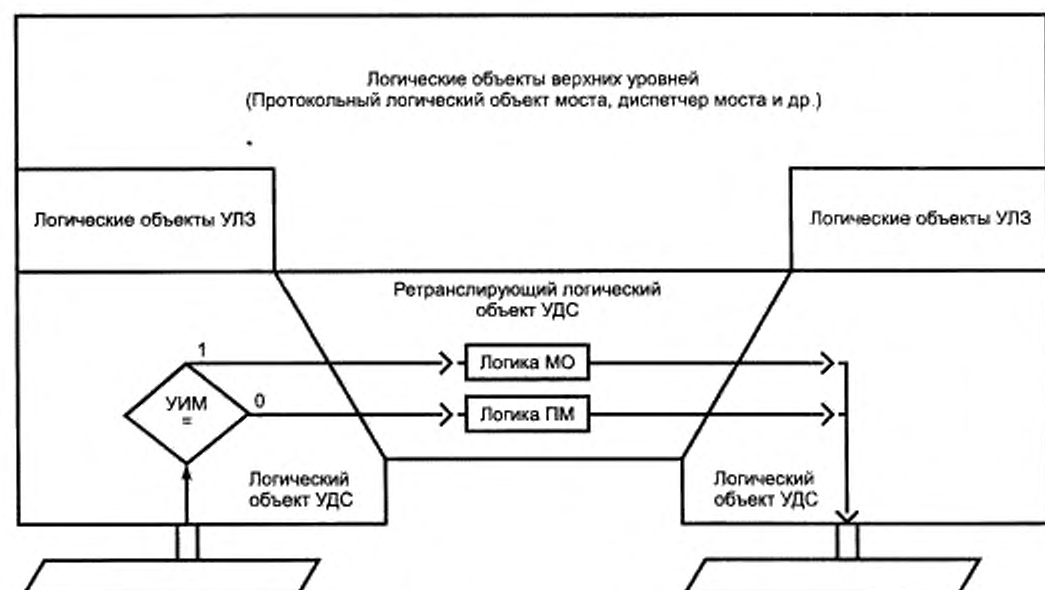
Рисунок С.1 — Логика операций моста ПМСО
