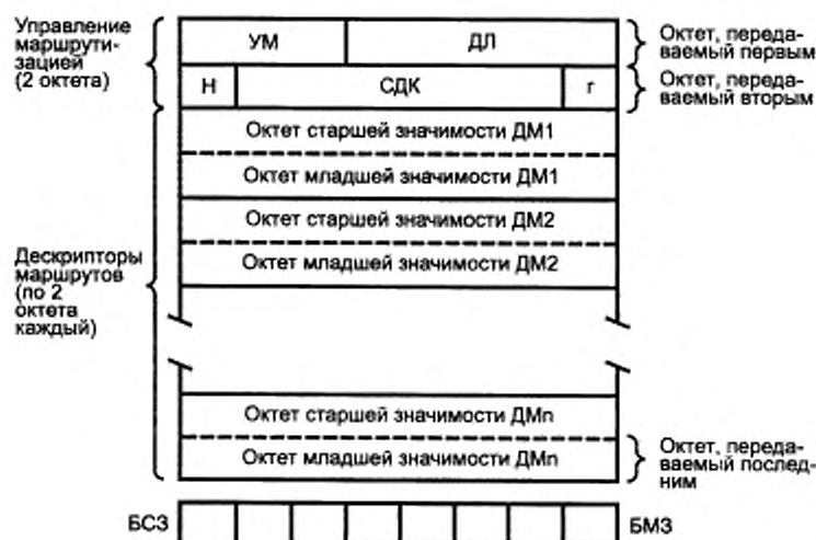
Рисунок С.3 — Поле информации маршрутизации
