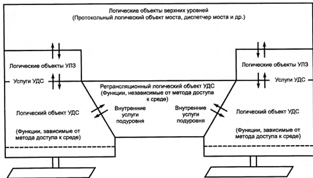
Рисунок 3.3 — Архитектура моста
