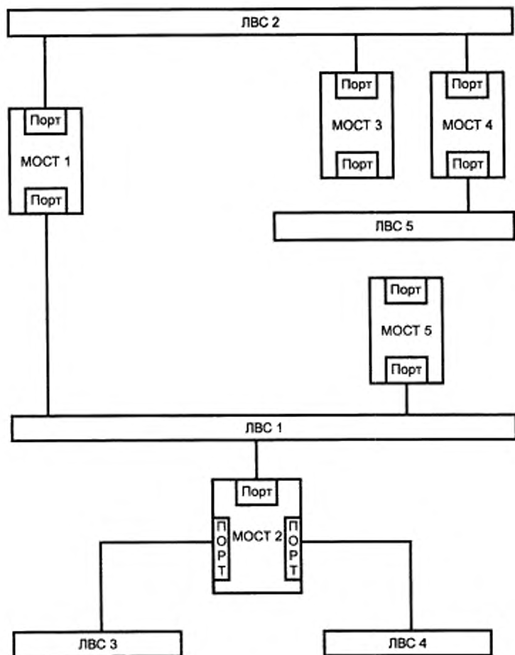
Рисунок 4.1 — Активная топология
