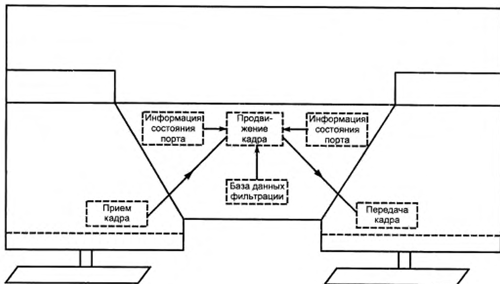
Рисунок 3.4 — Ретрансляция кадров УДС
