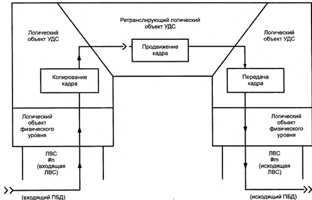
Рисунок С.2 — Элементы мостовой функции маршрутизации со стороны отправителя
