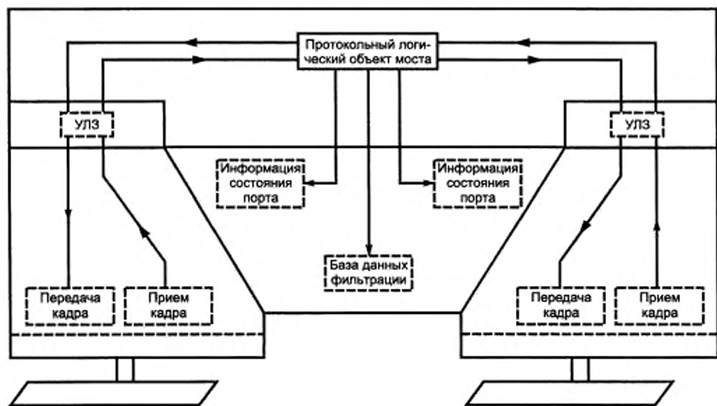
Рисунок 3.6 — Операции межмостового протокола
