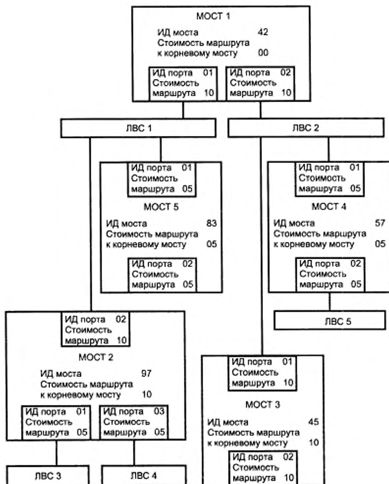
Рисунок 4.2 — Связующее дерево
