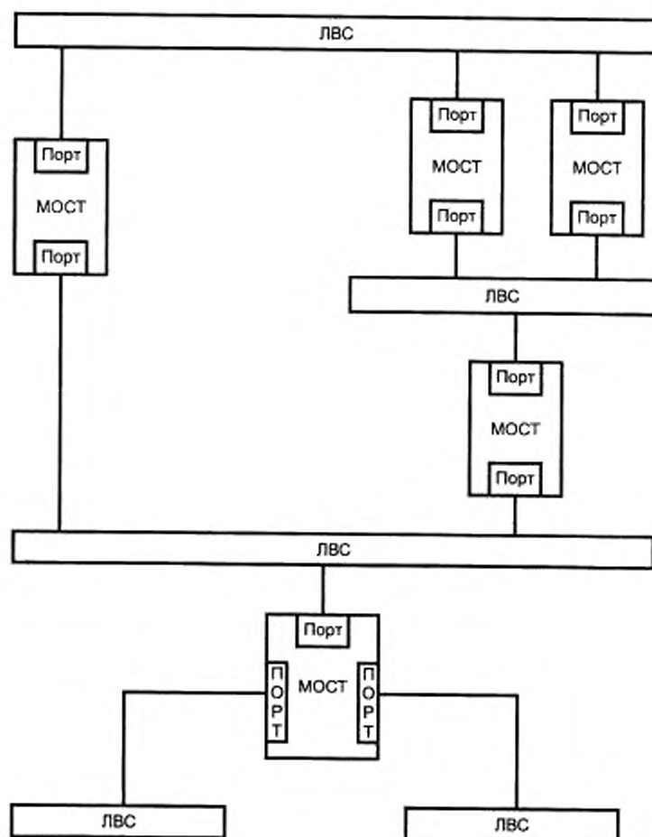
Рисунок 3.1 — Мостовая локальная вычислительная сеть
