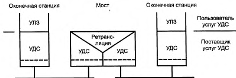
Рисунок 2.1 — Внутренняя организация подуровня УДС
