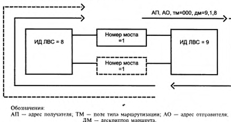
Рисунок С.8 — Иллюстрация проверки дублирования номера моста
