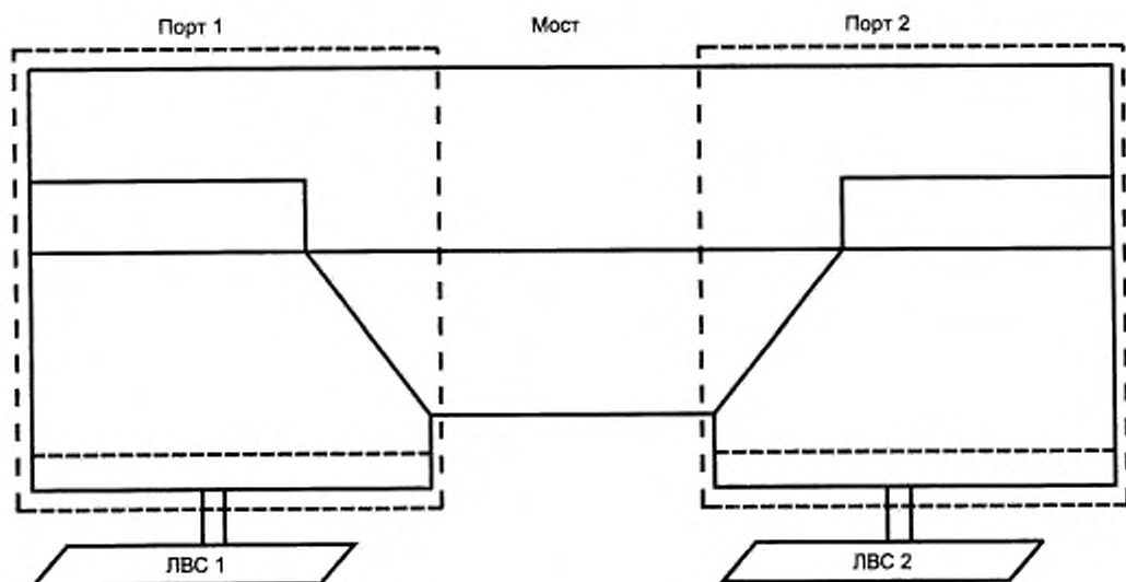
Рисунок 3.2 — Порты моста
