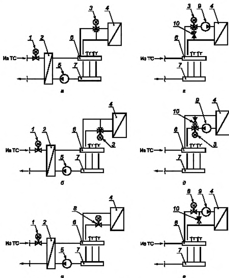
а, б, в — при независимом присоединении, г, д, е — при зависимом присоединении; 1 — внешний регулирующий клапан системы теплоснабжения вентиляции; 2 — теплообменник системы теплоснабжения вентиляции; 3 — трехходовой регулирующий клапан воздухонагревателя; 4 — воздухонагреватель; 5 — циркуляционный насос системы теплоснабжения вентиляции; 6 и 7 — распределительный и сборный коллекторы системы теплоснабжения вентиляции соответственно (могут отсутствовать); 8 — двухходовой регулирующий клапан воздухонагревателя; 9 — смесительно-циркуляционный насос узла обвязки воздухонагревателя; 10 — обратный клапан, ТС — тепловая сеть
