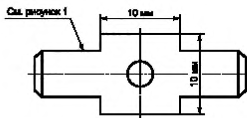
Рисунок 6 — Двухконцевой штекер (см. 8.3)
