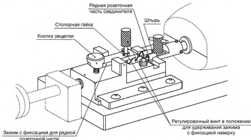
Рисунок В.5 — Регулировка оснастки
