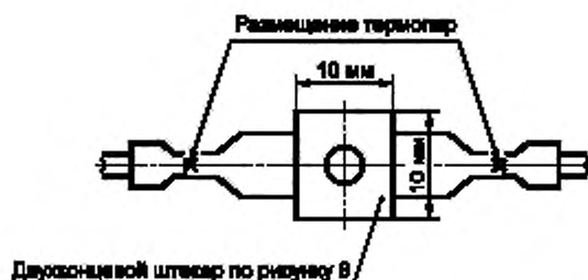
Рисунок 7 — Размещение термодпар при испытаниях (см. 8.3)
