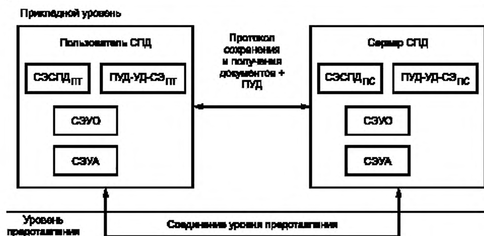
Рисунок 2 — Модель совместного использования СПД и ПУД
