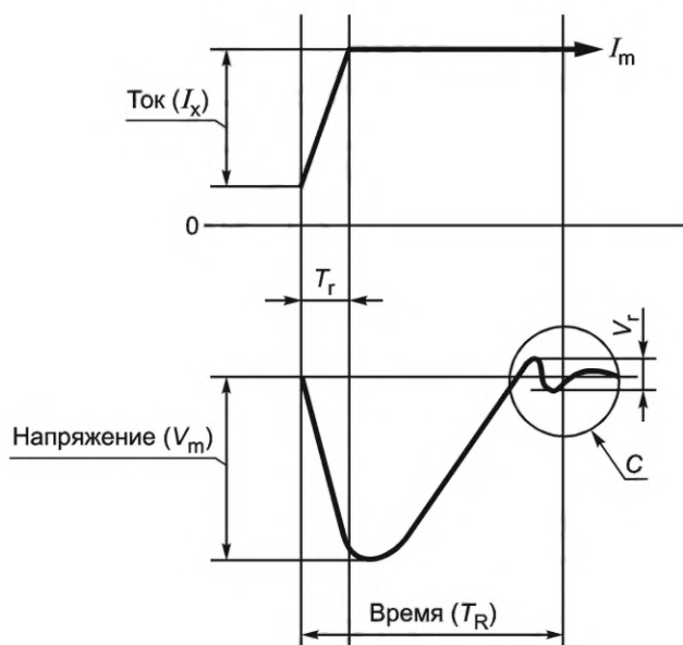
Рисунок 1 — Временная диаграмма переходного процесса при активной нагрузке
