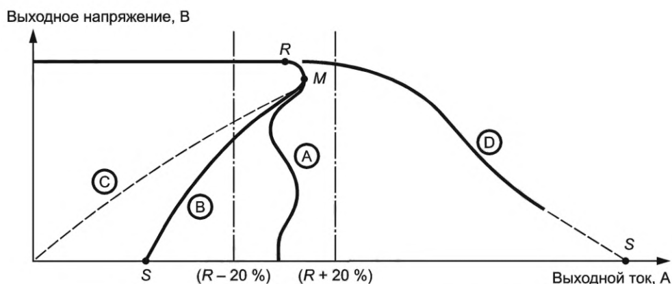
Рисунок С.1 — Защита от сверхтоков. Характеристики
