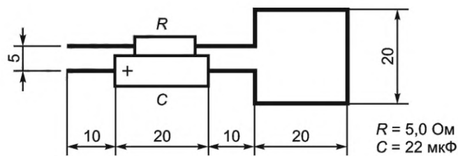
Рисунок А.3 — Схема подключения датчика тока
