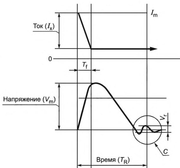
Рисунок 2 — Временная диаграмма переходного процесса без активной нагрузки
