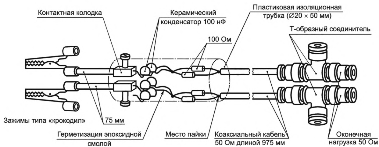
Рисунок А.1 — Дифференциальный пробник
