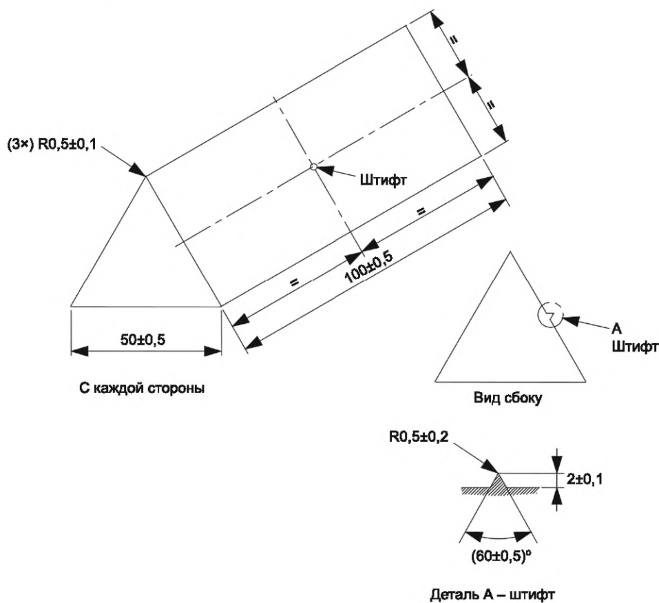
Рисунок 101 — Оправка
