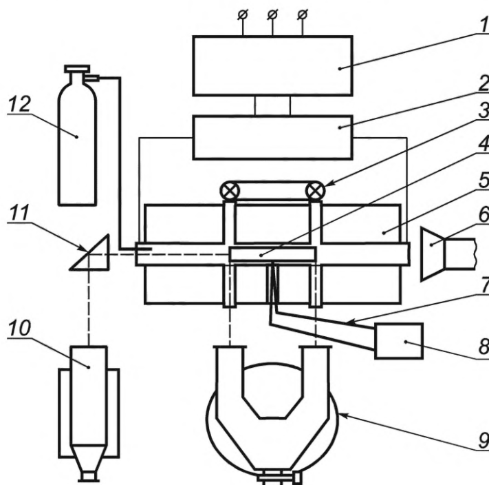
1 — автотрансформатор; 2 — силовой трансформатор; 3 — подсветка; 4 — испытываемый образец; 5 — печь дилатометра; 6 — вентиляционный отсос; 7 — термопара; 8 — измеритель ЭДС термопары; 9 — микроскоп-компаратор; 10 — пирометр; 11 — призма полного внутреннего отражения; 12 — баллон с инертным газом
