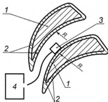
1 — лопатка; 2 — никелевая фольга; 3 — датчик (преобразователь) толщиномера; 4 — толщиномер
