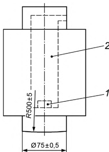
1 — акселерометр; 2 — камера для установки акселерометра
