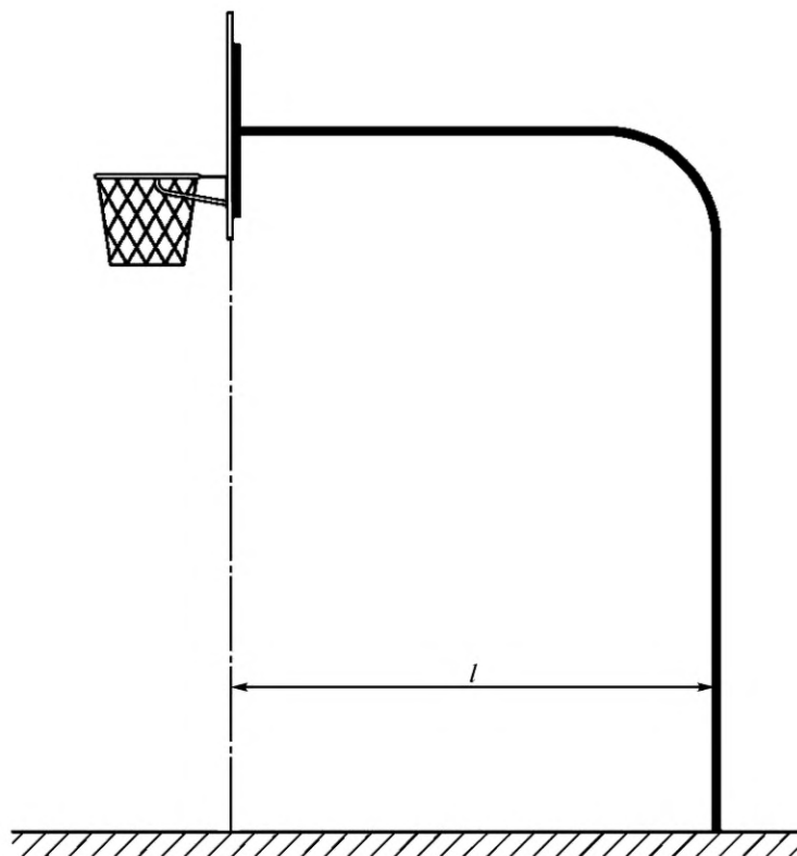
Рисунок 1 — Пример свободного пространства под щитом
