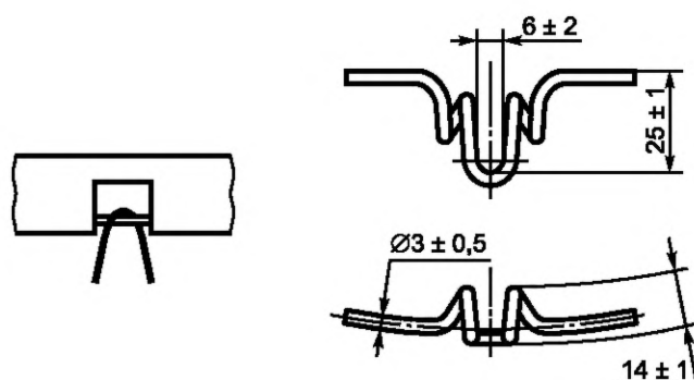
Рисунок 6 — Пример крючков для крепления сетки
