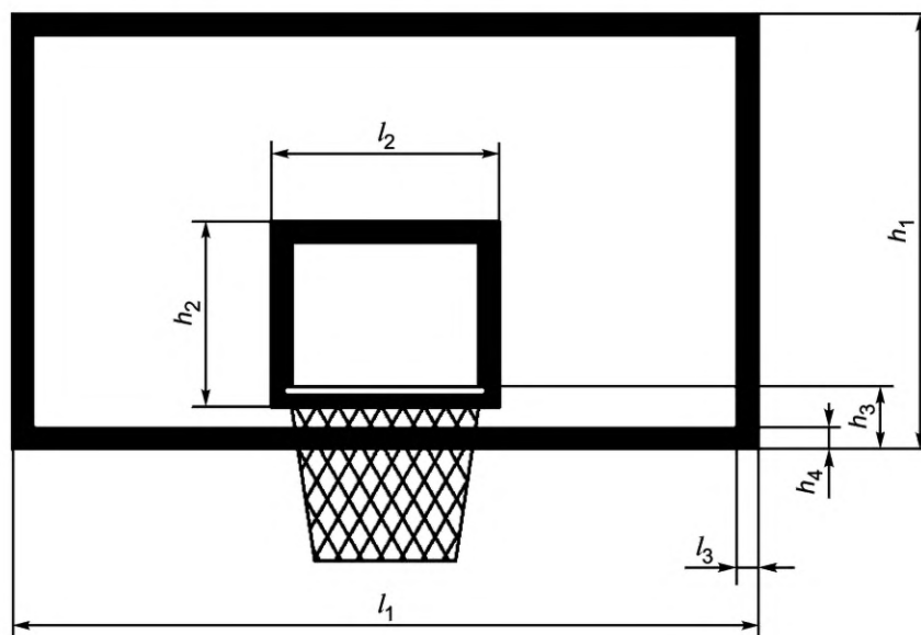
Рисунок 3 — Размеры и разметка баскетбольного щита
