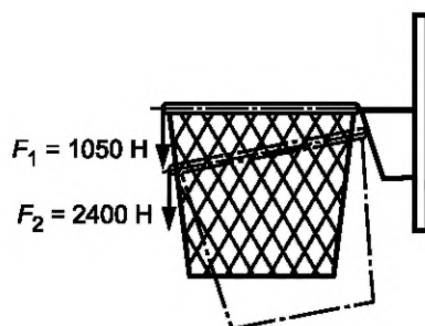
Рисунок Б.2 — Схема приложения нагрузки при испытании кольца с амортизатором двумя нагрузками
