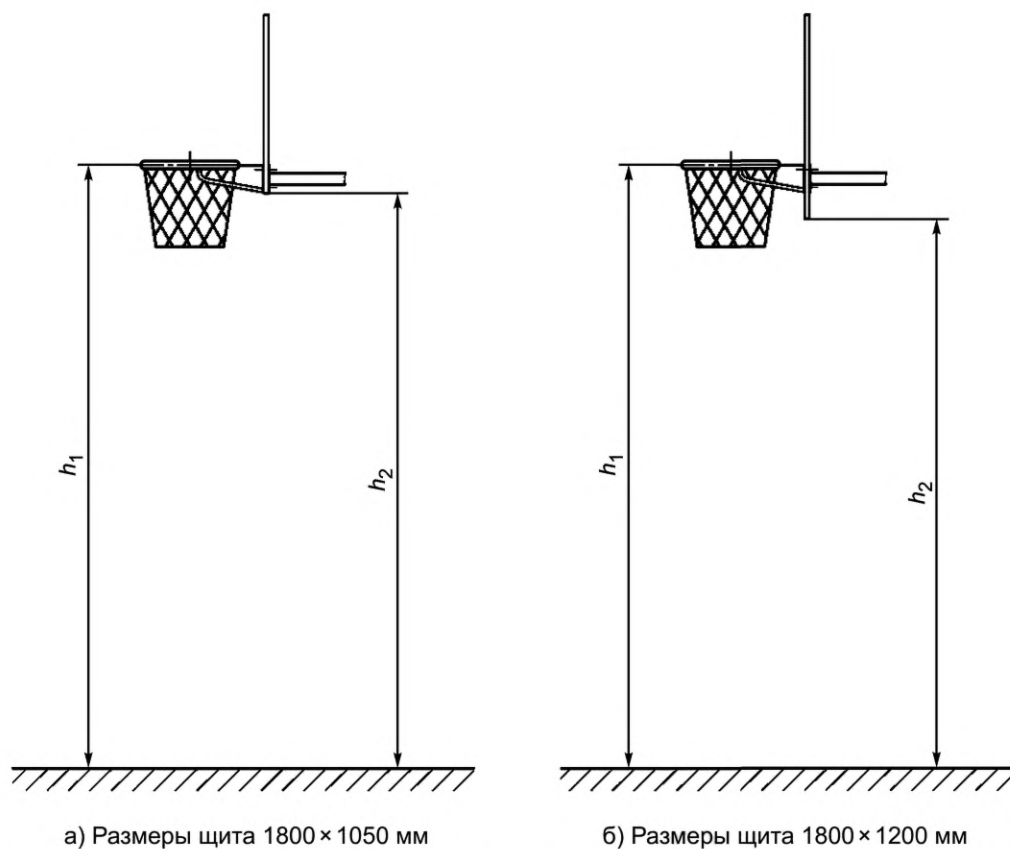
Рисунок 2 — Высота установки корзины для баскетбольного оборудования классов А—D
