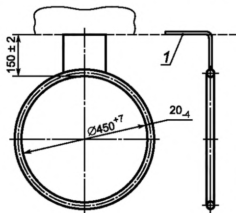
Рисунок 5 — Размеры баскетбольного кольца
