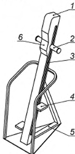
1 — дисплей; 2 — подвижная ручка; 3 — направляющая; 4 — платформа; 5 — базовая рама; 6 — регулятор сопротивления
