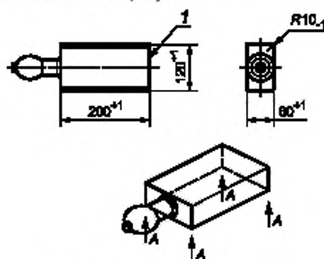
1 — передняя часть; А — точки опирания для измерения минимального зазора 60 мм
