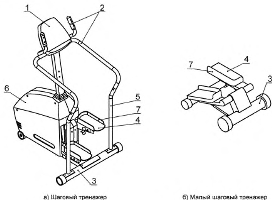
Рисунок 1 — Примеры шаговых тренажеров
