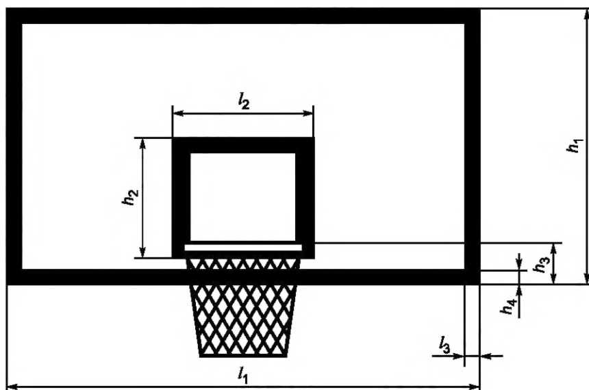
Рисунок 8 — Рекомендуемые размеры баскетбольного щита и размеры маркировки
