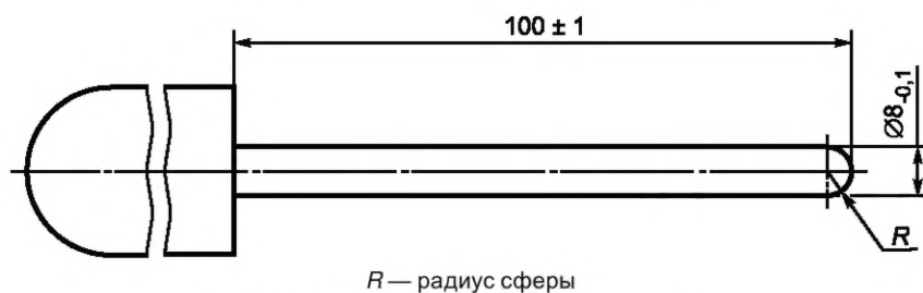
Рисунок Г.1 — Стержень-палец А (малый)
