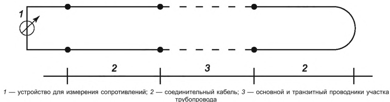
Рисунок 1 — Схема проведения испытания
