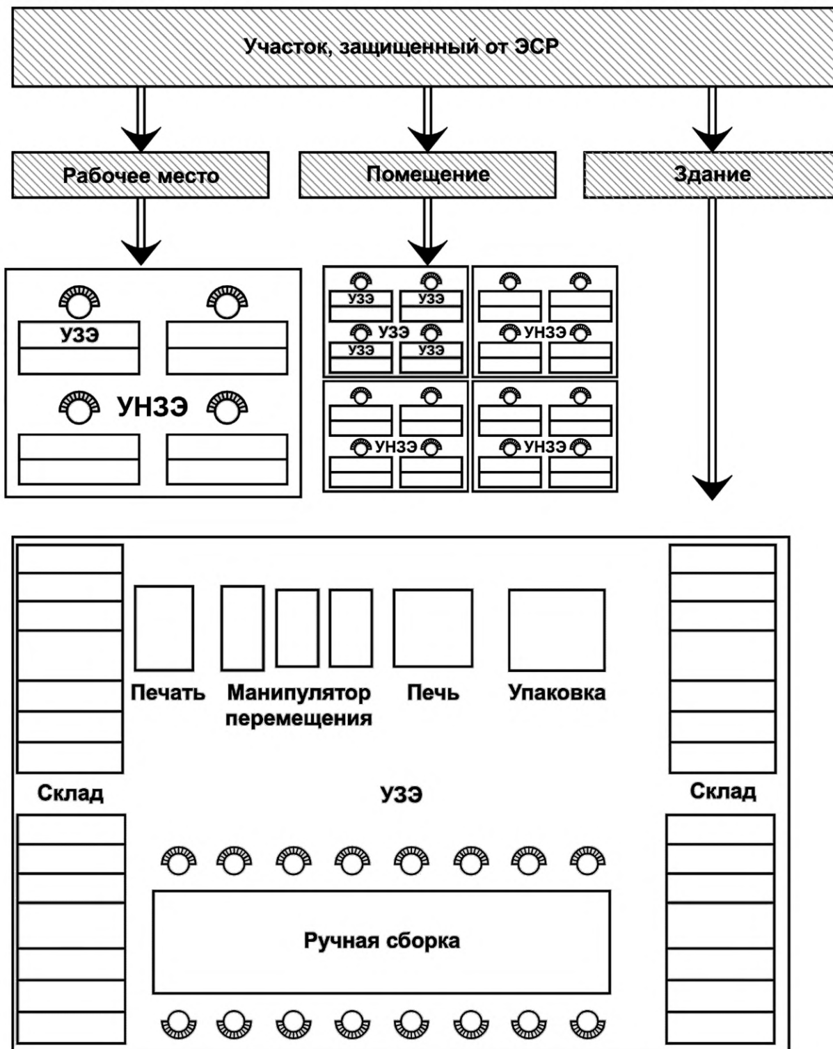
Рисунок А.1 — Пример схемы УЗЗ
