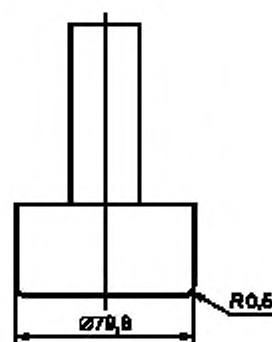
Рисунок 3 — Цилиндрический индентор
