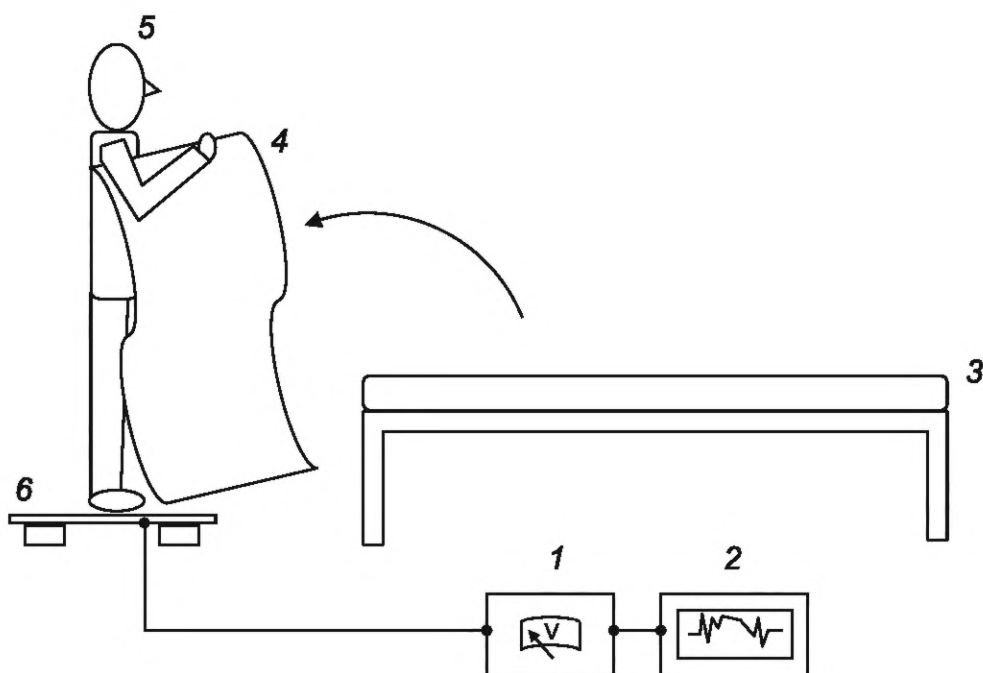
1 — электростатический вольтметр; 2 — записывающее устройство; 3 — кровать или смотровой/операционный стол; 4 — испытуемое постельное белье или хирургическая пленка; 5 — оператор, без обуви; 6 — металлическая подставка на изоляционном основании, сопротивление между металлической площадкой и заземлением более 10^{13} Ом
