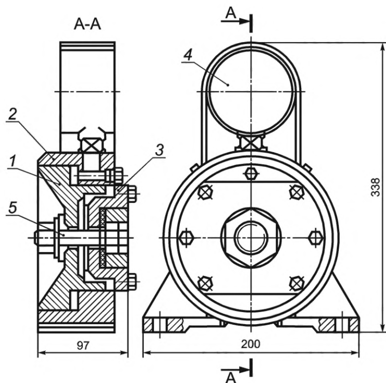
Рисунок В.1 — Общий вид устройства УТБ-40
