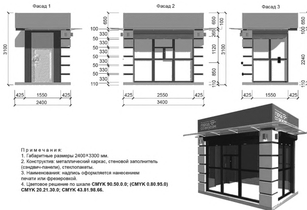
Рисунок А.9 — Киоск 3,4×2,4 м
