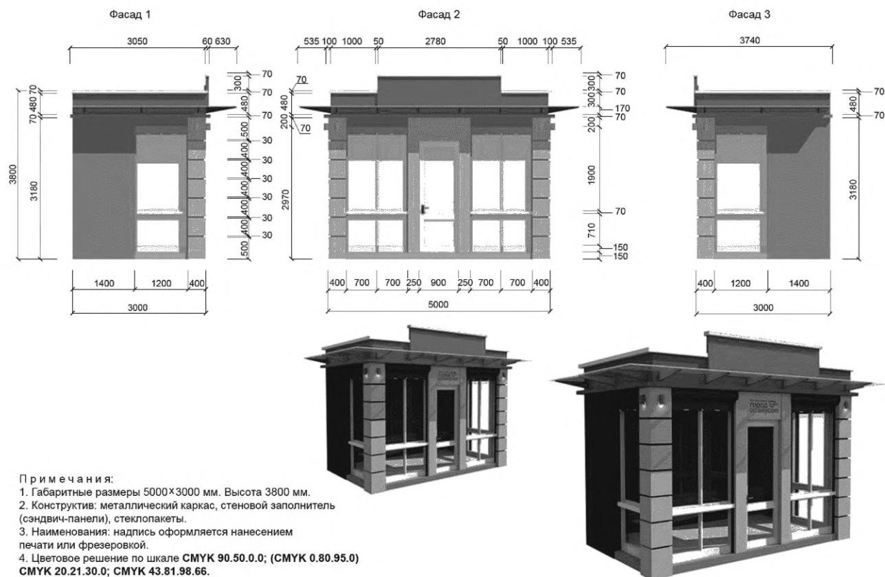
Рисунок А.10 — Павильон 5х3 м
