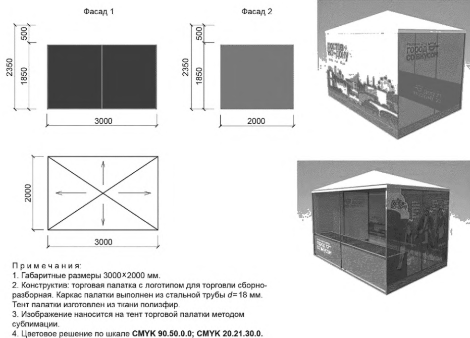
Рисунок А.4 — Палатка 2×3 м
