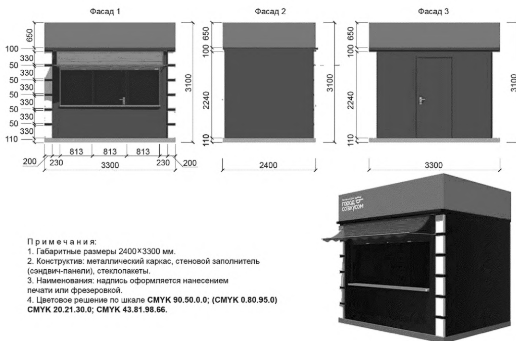
Рисунок А.5 — Киоск 3,3×2,4 м
