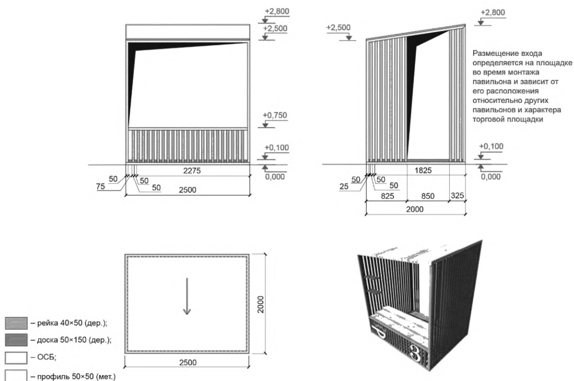
Рисунок А.7 — Павильон 2,5×2 м, тип 3
