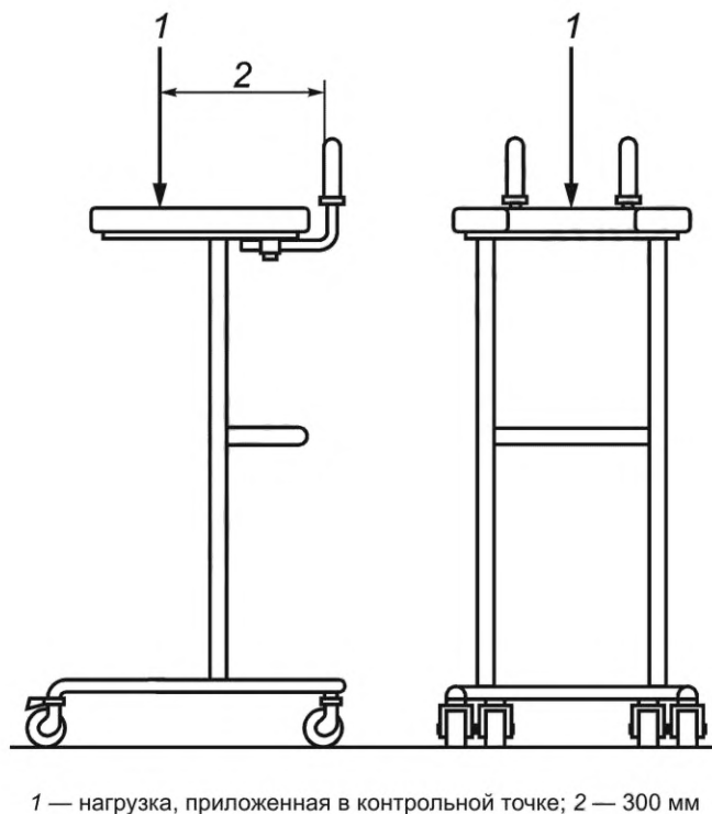
Рисунок 12 — Схема нагружения при испытаниях на статическую и усталостную прочность
