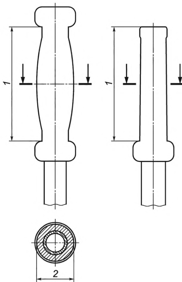
Рисунок 5 — Элементы рукоятки
