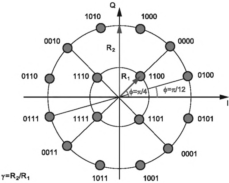
Рисунок 11 — Отображение битов на созвездие 16APSK
