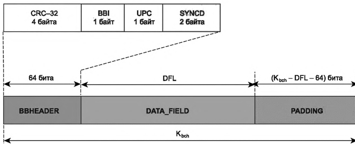
Рисунок 3 — Формат кадра базовой полосы на выходе ПАР
