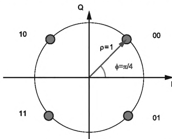
Рисунок 9 — Отображение битов на созвездие QPSK
