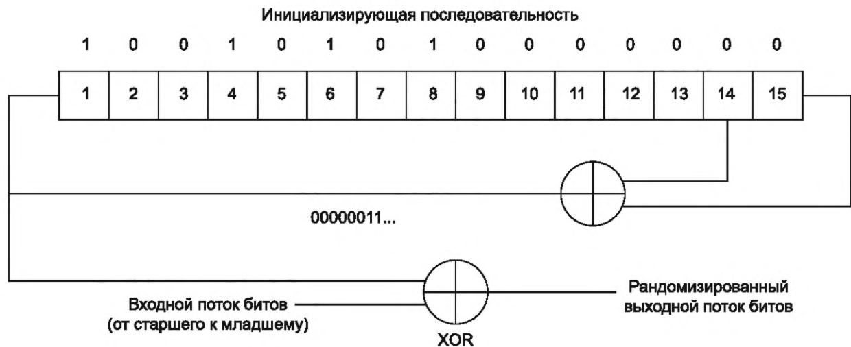
Рисунок 4 — Схема рандомизации данных
