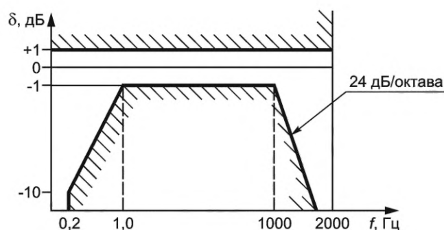
Рисунок А.4 — Амплитудно-частотная характеристика измерительной системы
