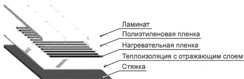
Рисунок Е.3 — Слои пола при установке нагревательной секции на основе нагревательной пленки
