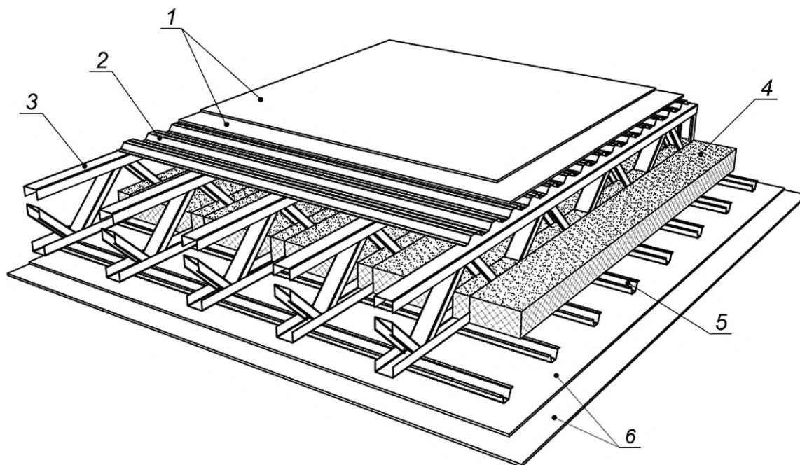
1 — верхняя обшивка; 2 — профилированный настил; 3 — фермы каркаса КОП; 4 — звукоизоляционный слой; 5 — стальные профили обрешетки; 6 — нижняя обшивка
