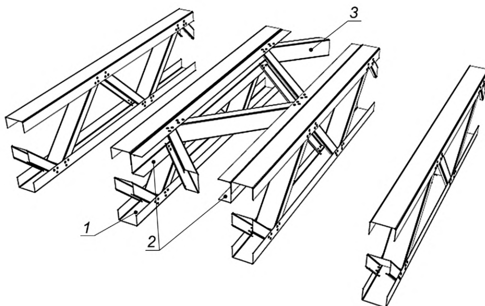
1 — фермы каркаса КОП; 2 — опорные профили; 3 — связи из холодногнутых профилей С-образного сечения
