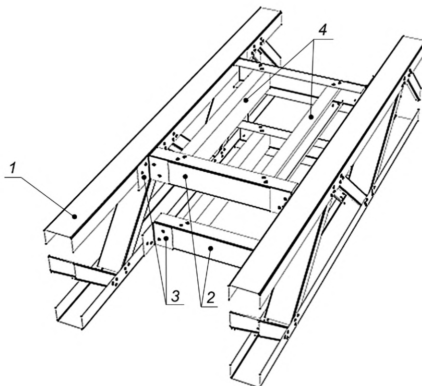
Рисунок В.4 — Схема обрамления проема в КОП с каркасом из ферм
