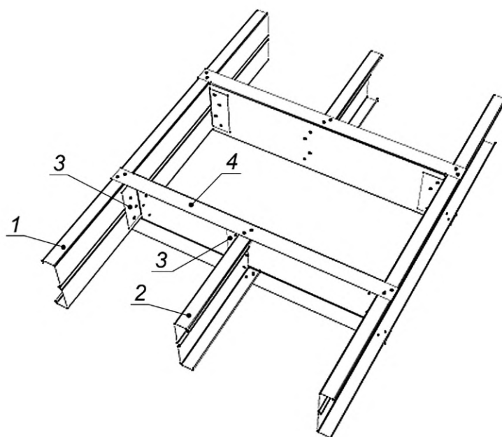
Рисунок В.3 — Схема обрамления проема большого размера в КОП с каркасом из балок
