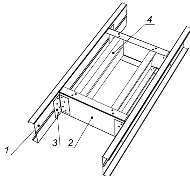
Рисунок В.1 — Схема обрамления проема в КОП с каркасом из балок с устройством направляющей
