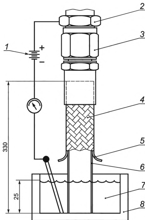
1 — источник питания постоянного тока; 2 — электрод 2; 3 — гайка фитинга; 4 — оплетка шланга; 5 — оголенная оплетка; 6 — ПТФЕ трубка; 7 — электрод 1; 8 — диэлектрический контейнер
