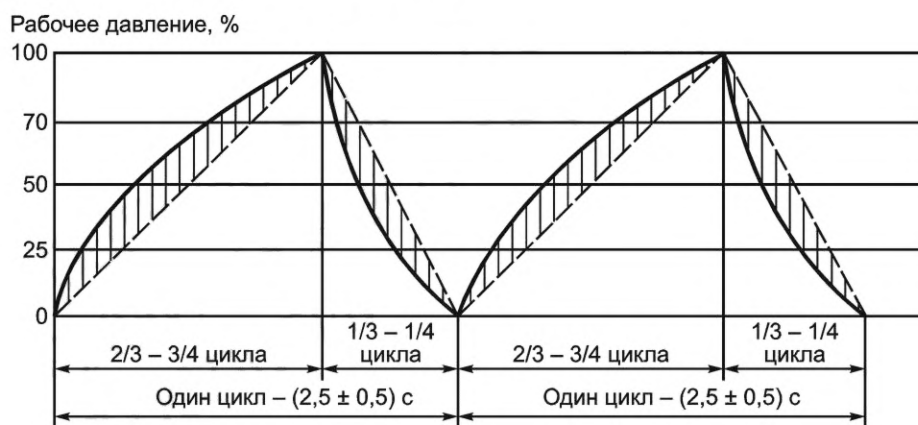
Рисунок 2 — График испытания
