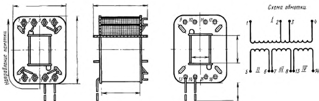
Данные обмоток
