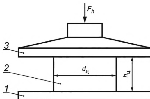
1 — столик прибора; 2 — проба мякиша; 3 — индентор-поршень диаметром 49 мм; d_{\text{ц}} — диаметр цилиндрической пробы, равный 36 мм; h_{\text{ц}} — высота цилиндрической пробы, равная 20 мм
