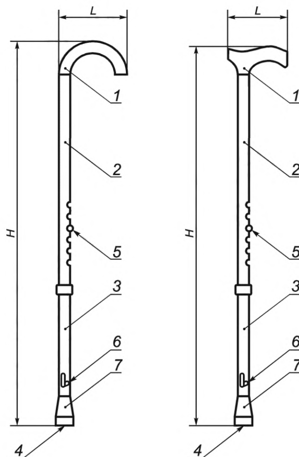
1 — рукоятка; 2 — верхняя секция стойки; 3 — нижняя секция стойки; 4 — устройство противоскольжения; 5 — фиксатор регулирования длины стойки; 6 — фиксатор устройства противоскольжения; 7 — наконечник; H — высота трости; L — длина рукоятки
