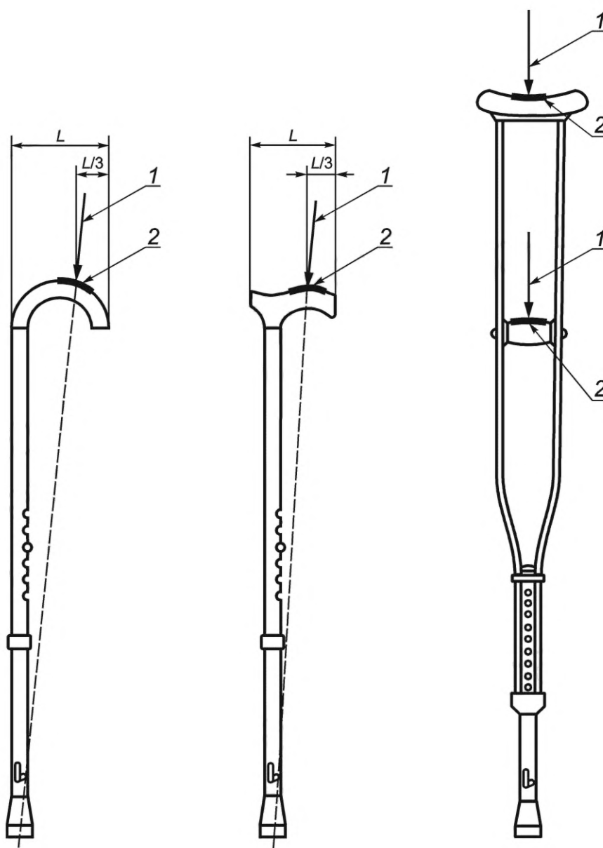
Рисунок 3 — Испытание изделий на прочность
