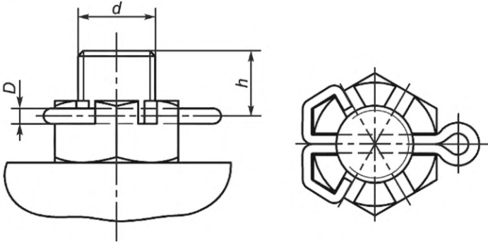
Рисунок 1 — Расположение отверстий под шплинты
