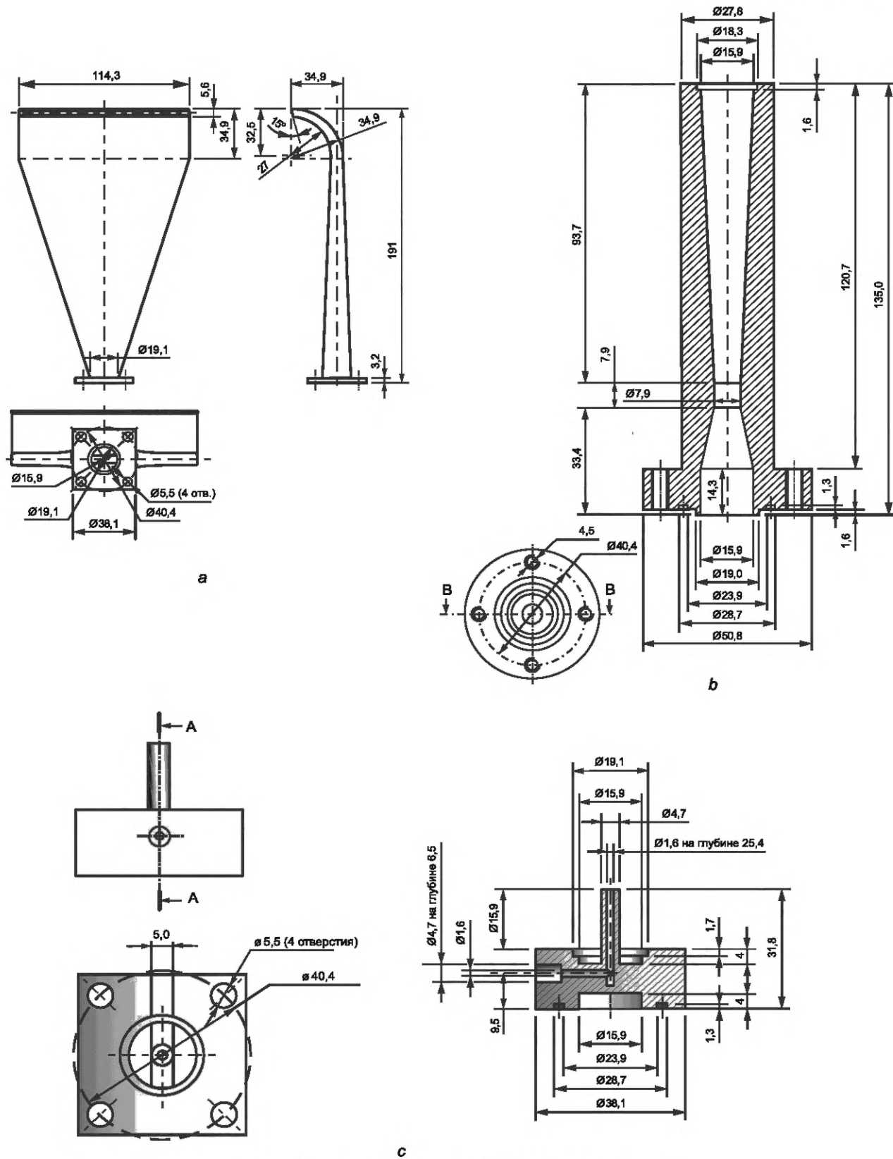
Рисунок 2 — Пылезаборная трубка, трубка Вентури и эжектор
