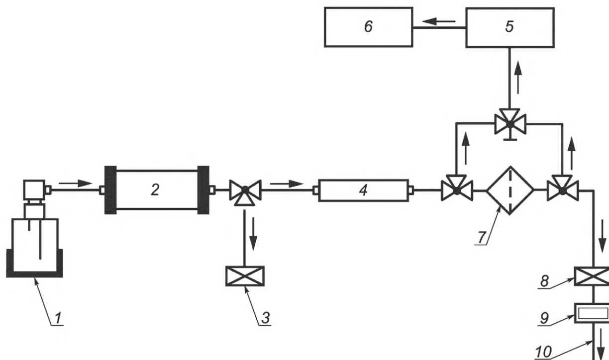
1 — распылитель; 2 — диффузионный осушитель; 3 — клапан сброса давления с НЕРА-фильтром в линии; 4 — нейтрализатор; 5 — КДЭП; 6 — КСЧ; 7 — фильтродержатель; 8 — НЕРА-фильтр на выпускной линии; 9 — блок контроля расхода воздуха; 10 — вакуумированная линия
