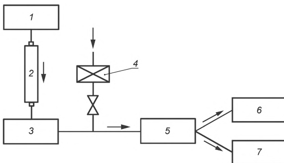
1 — генератор аэрозоля; 2 — нейтрализатор; 3 — КДЭП; 4 — воздух, пропущенный через HEPA-фильтр; 5 — разделитель потока; 6 — аэрозольный электрометр/поверенный КСЧ; 7 — испытуемый КСЧ
