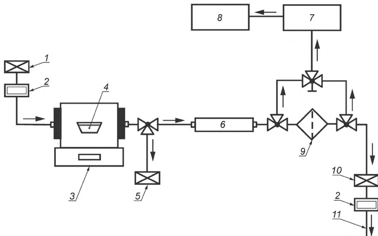
Рисунок 2 — Схема испытательного стенда для проведения испытаний с полидисперсным аэрозолем для определения фракционной (зависящей от размера частиц) эффективности улавливания
