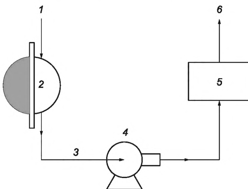
1 — подача чистой среды-носителя; 2 — секция для среды-носителя; 3 — отбор проб среды-носителя; 4 — побудитель расхода; 5 — аналитический детектор; 6 — сброс
